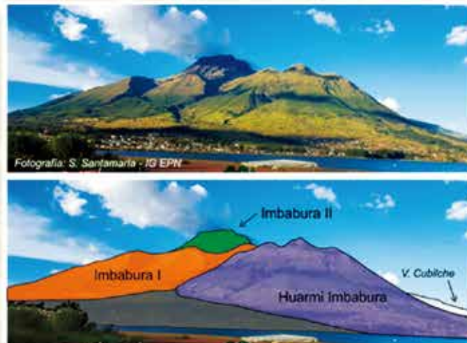
Figura 1. Vista panorámica norte del Complejo volcánico Imbabura - Cubilche
